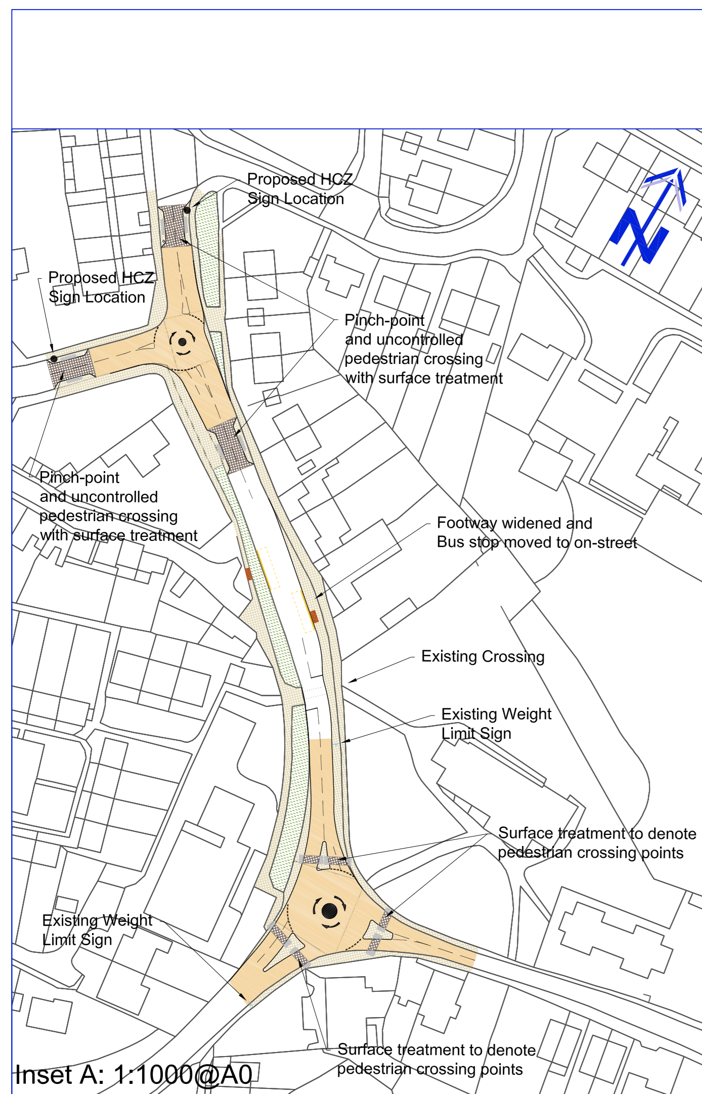
Inset A: 1:1000@A0
